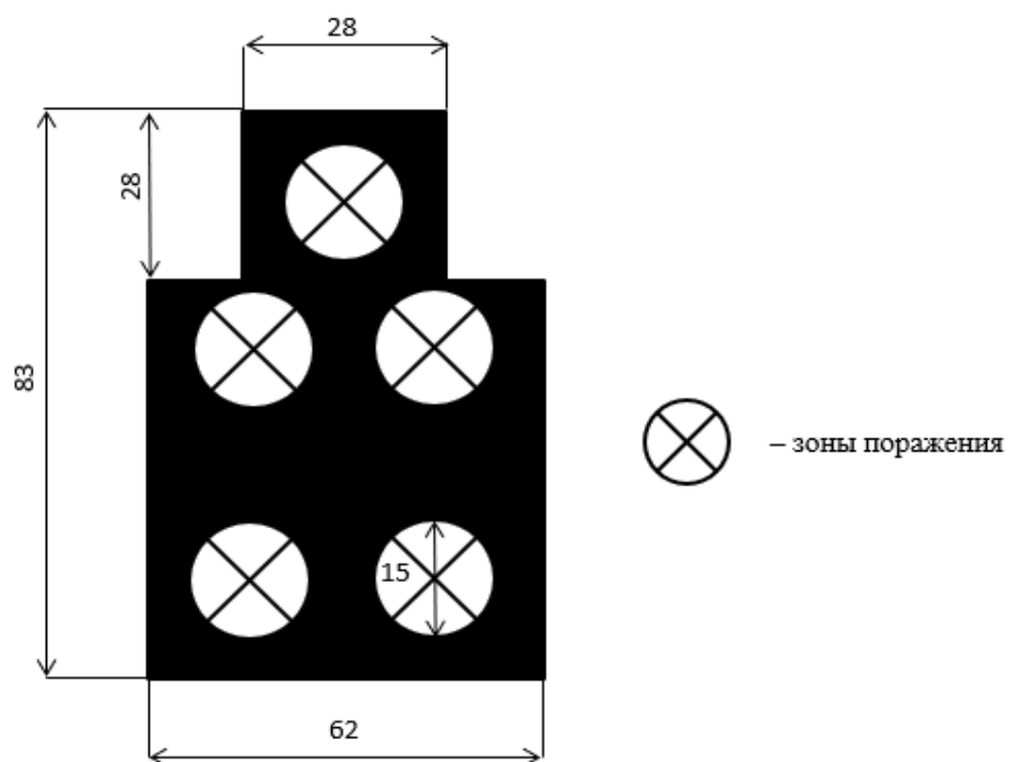
№ 3 – неметаллическая мишенная установка «Поясная фигура» (размеры указаны в см)
