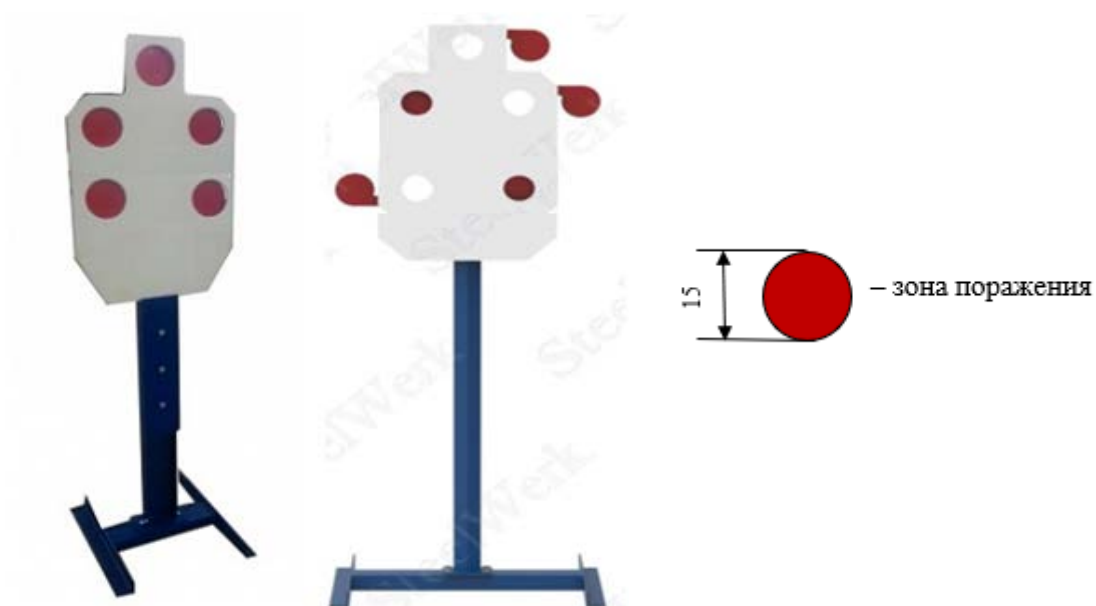
№ 2 – металлическая мишенная установка стандарта IPSC «Гонг метрический D с 5 зонами поражения»* (размеры указаны в см, габариты)
