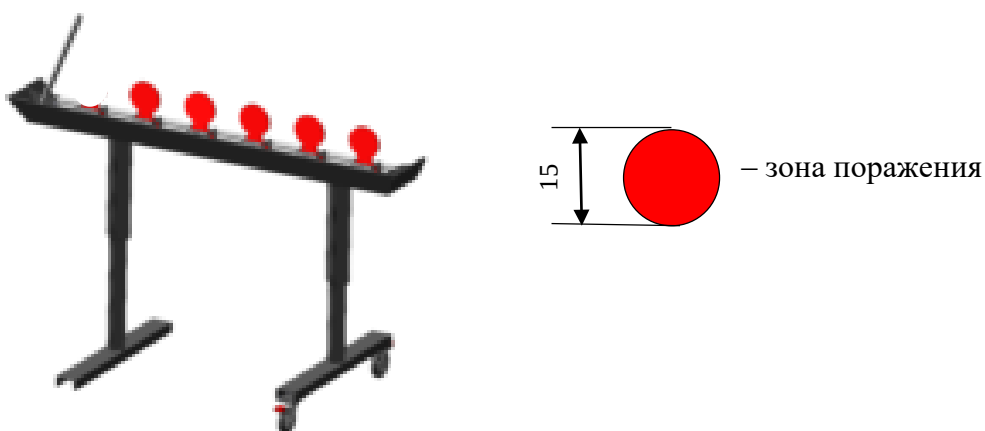
№ 2 – металлическая мишенная установка стандарта IPSC «Гонг метрический D с 5 зонами поражения»* (размеры указаны в см, габариты)
