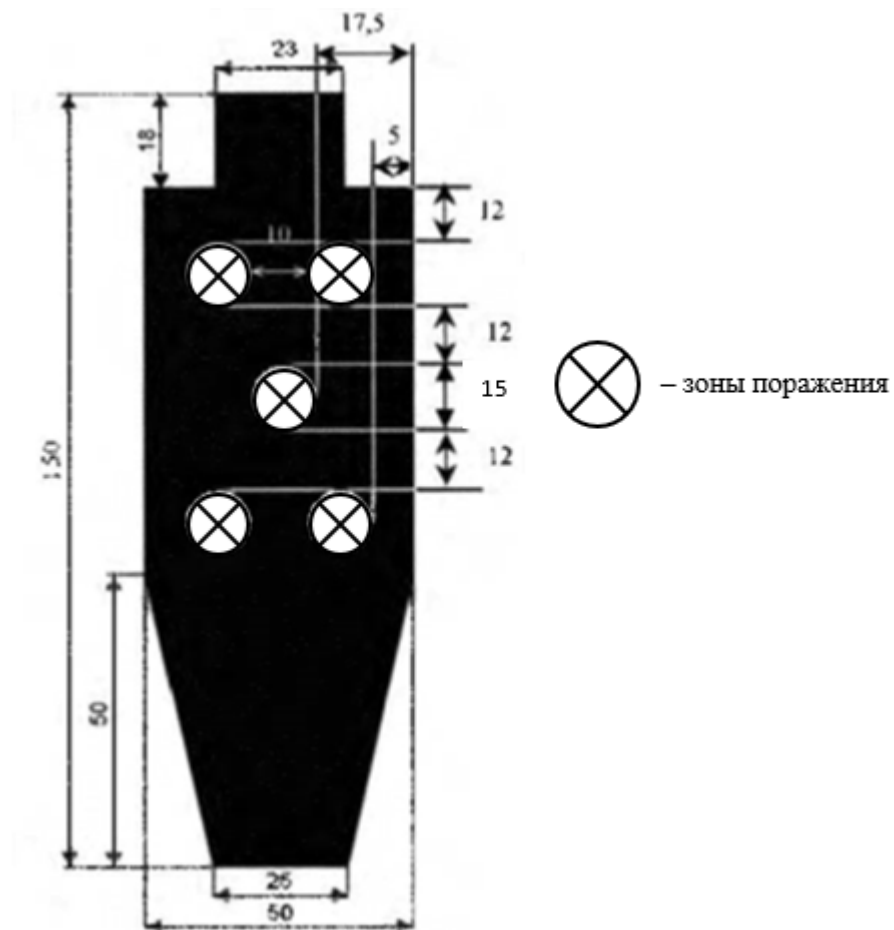
№ 4 – неметаллическая мишенная установка «Ростовая фигура» (размеры указаны в см)
