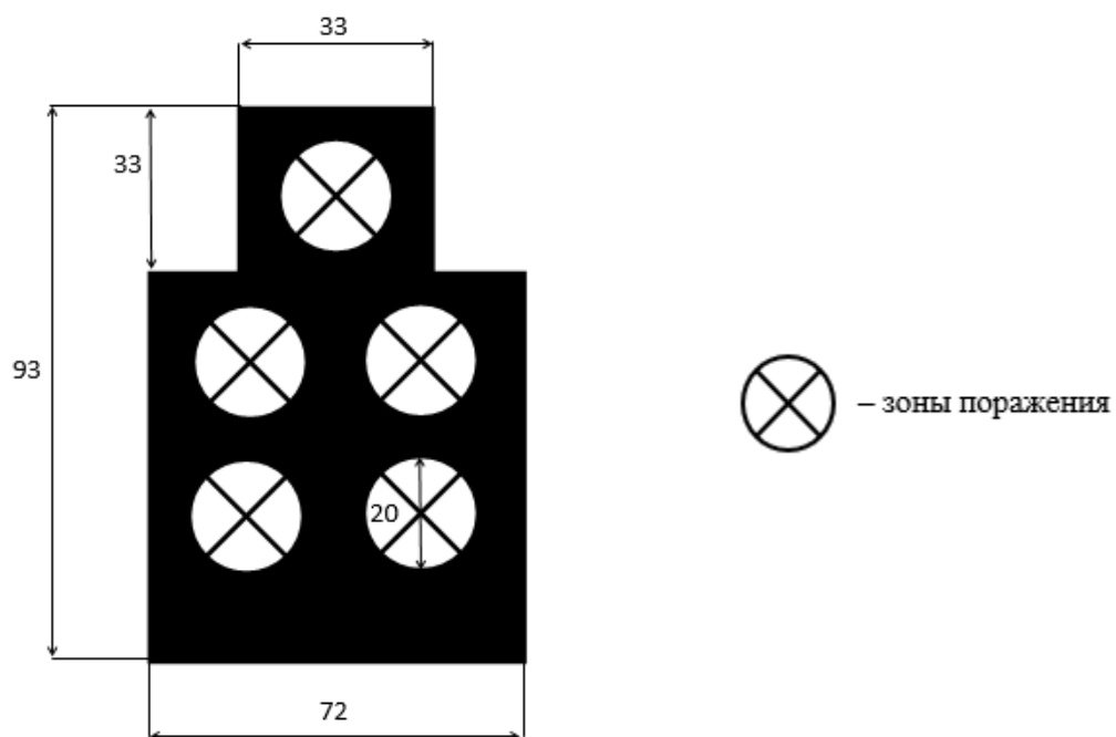
№ 7 – неметаллическая мишенная установка «Поясная фигура» (размеры указаны в см)
